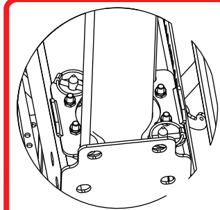
SISTEM DE FIXARE RAPIDĂ A CILINDRULUI
