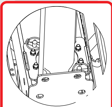
SISTEM DE FIXARE RAPIDĂ A CILINDRULUI
